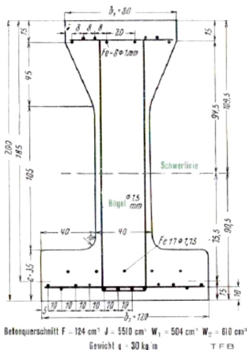
Section d'une poutre Hoyer armée de fils d'acier précontraints
